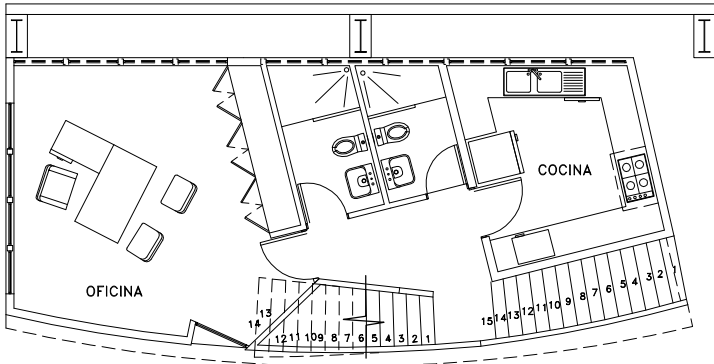
PLANTA SEGUNDO PISO
